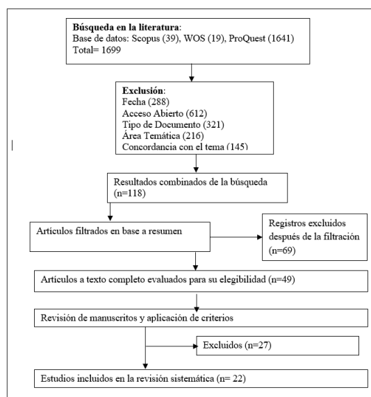
Figura 1: Flujo de selección de artículos.
